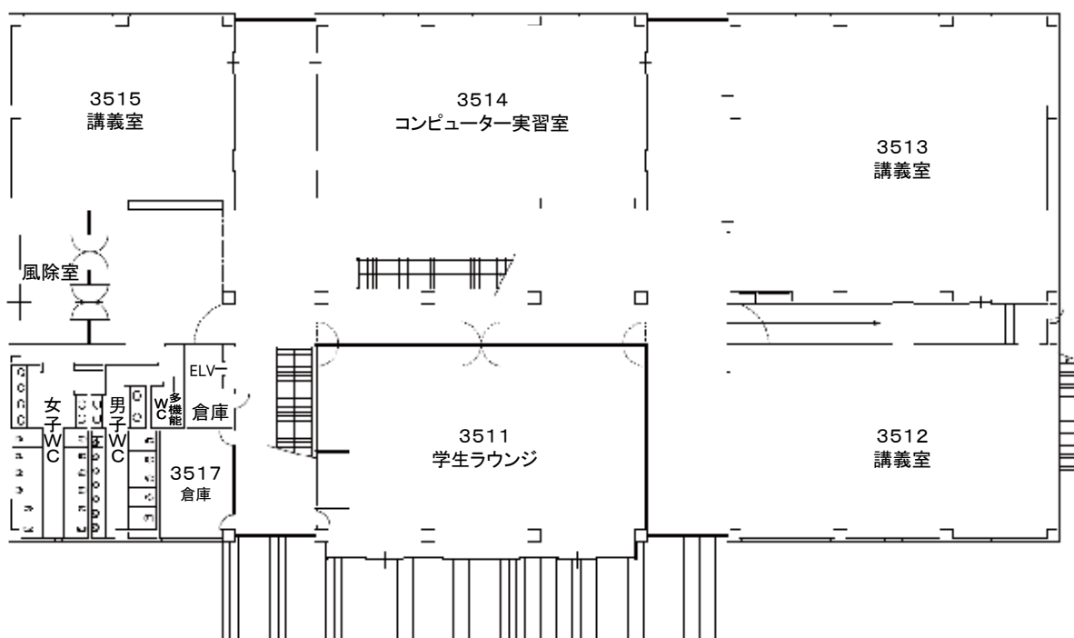
1階 平面図
