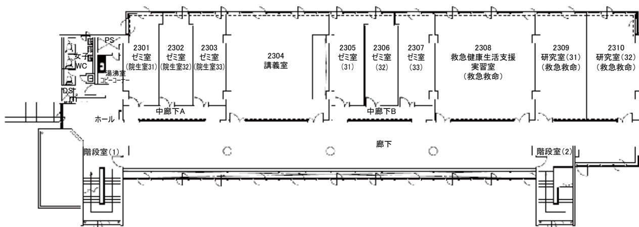
3階 平面図
