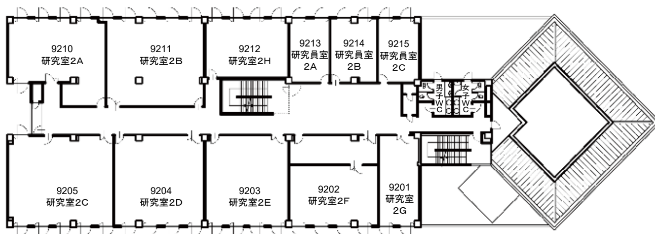
2階 平面図
