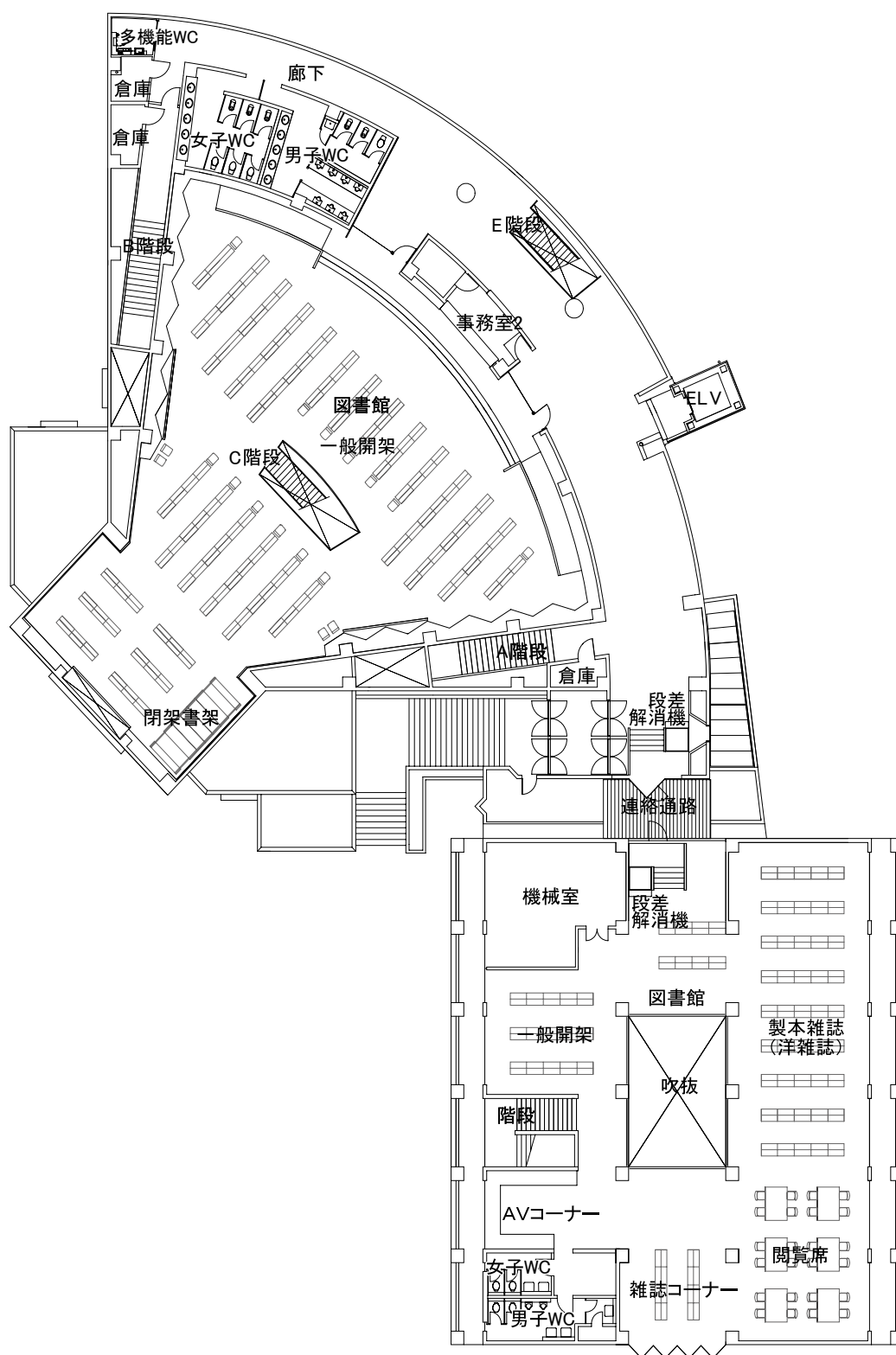
2階 平面図
