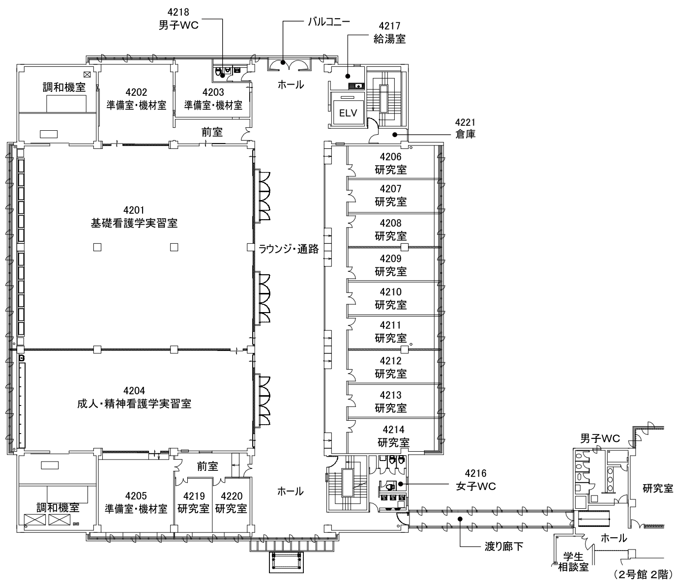
2階 平面図
