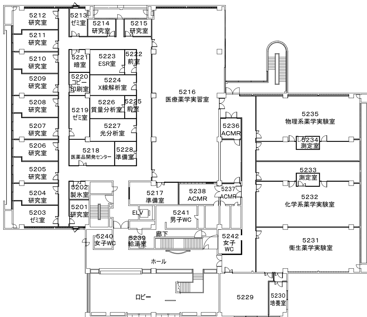
2階 平面図
