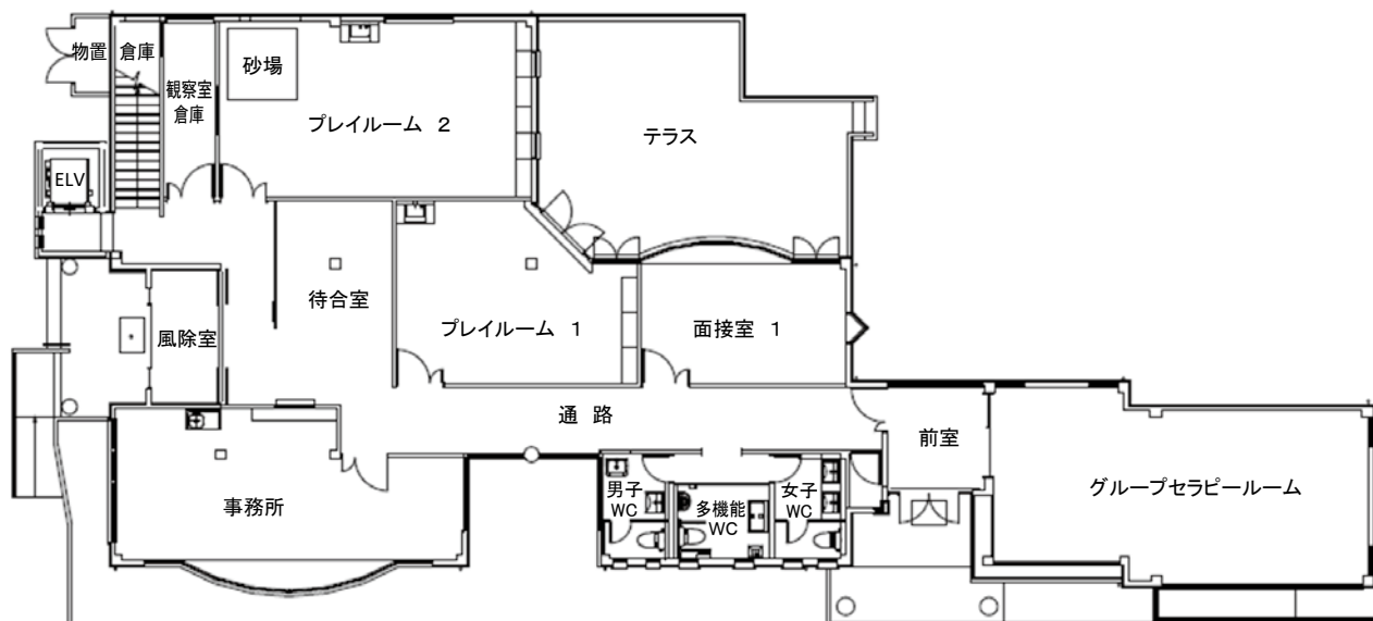
1階 平面図
