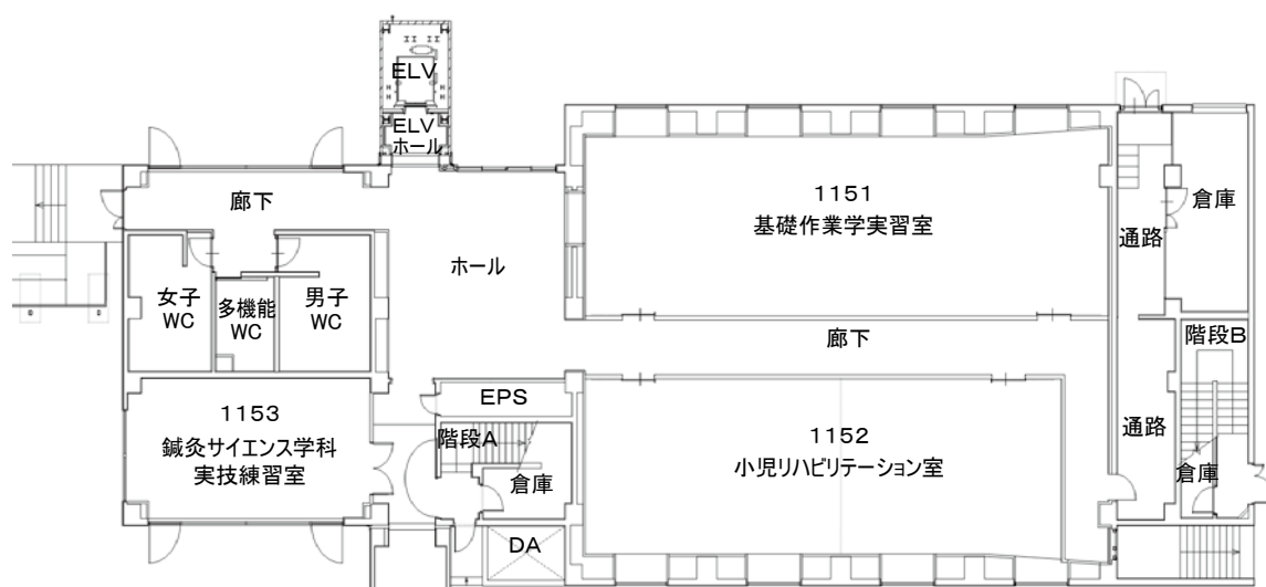
新館 1 階 平面図
